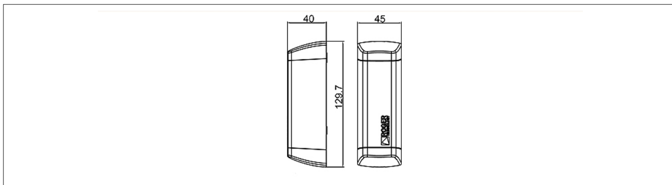
DIMENSIONS
